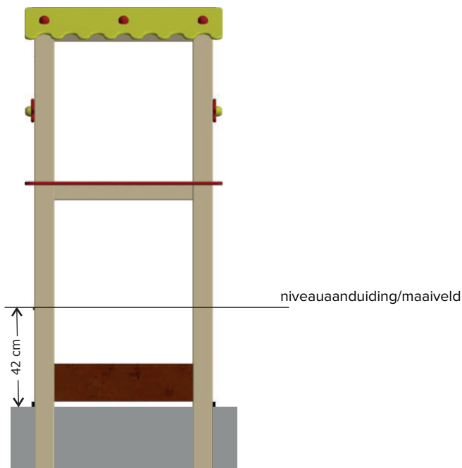
Plaatsing in zandbak of schorslaag (los bodemmateriaal)
