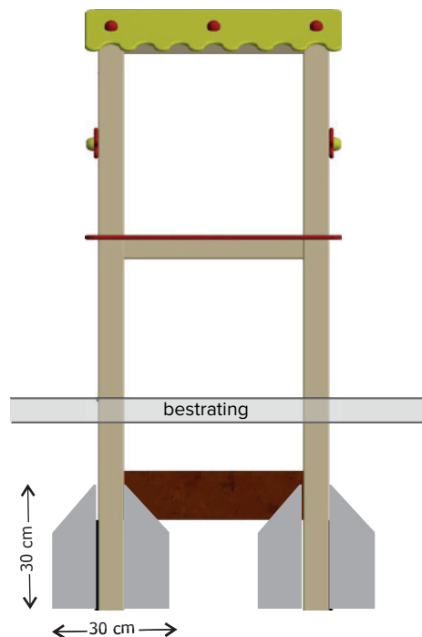
Plaatsing in bestrating of rubber tegels (vast bodemmateriaal)
