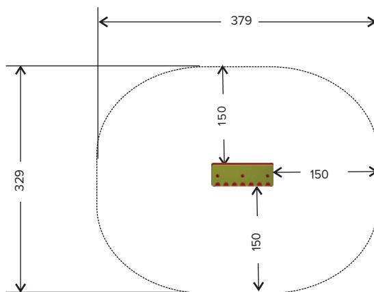
Plaatsing in bestrating of rubber tegels (vast bodemmateriaal)
