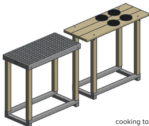
sieve table +/- 33,5 kg
