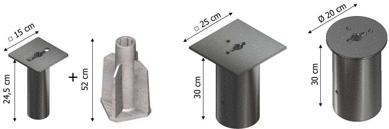
Type 1 grondkoker + bijhorende paalvoet voor losse grond bovenplaat vierkant 15cm
